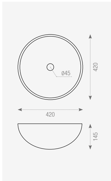
186490 Lavabo Pan De Plata 42×42×14,5 cm./16.5"×16.5"×5.7" E200
