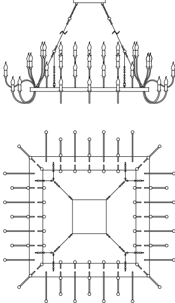
Item Moulin Rouge EX22 L.200 x D.200 cm H.210 cm
