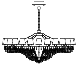
Item Ophelia EX07 Ø 146 cm H.124 cm min
