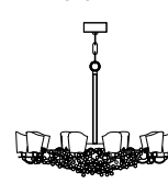
Item PG402 - 416/420 Ø 82 cm H.91 cm min
