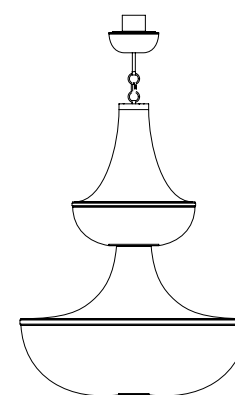
Item Margherita EX01 Ø 140 cm H.230 cm min
