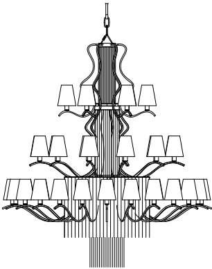
Item Sinuosa EX01 Ø 172 cm H. 230 cm min
