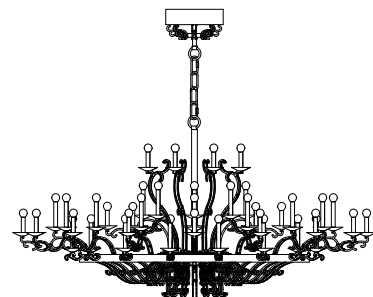
Item Morgana EX15 Ø 193 cm H.155 cm min
