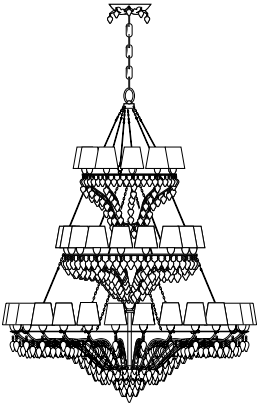
Item Ophelia EX01 Ø 146 cm H.280 cm min
