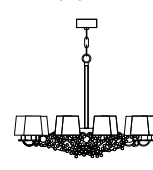
Item PG428/429 Ø 82 cm H.91 cm min
